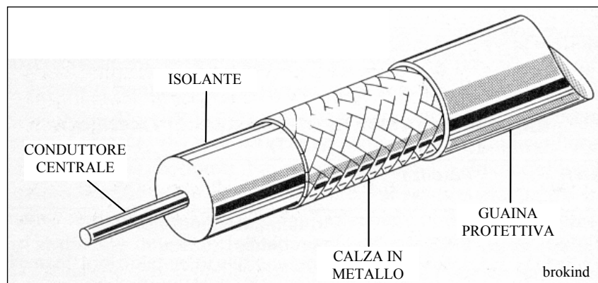
Spaccato di un cavo coassiale
